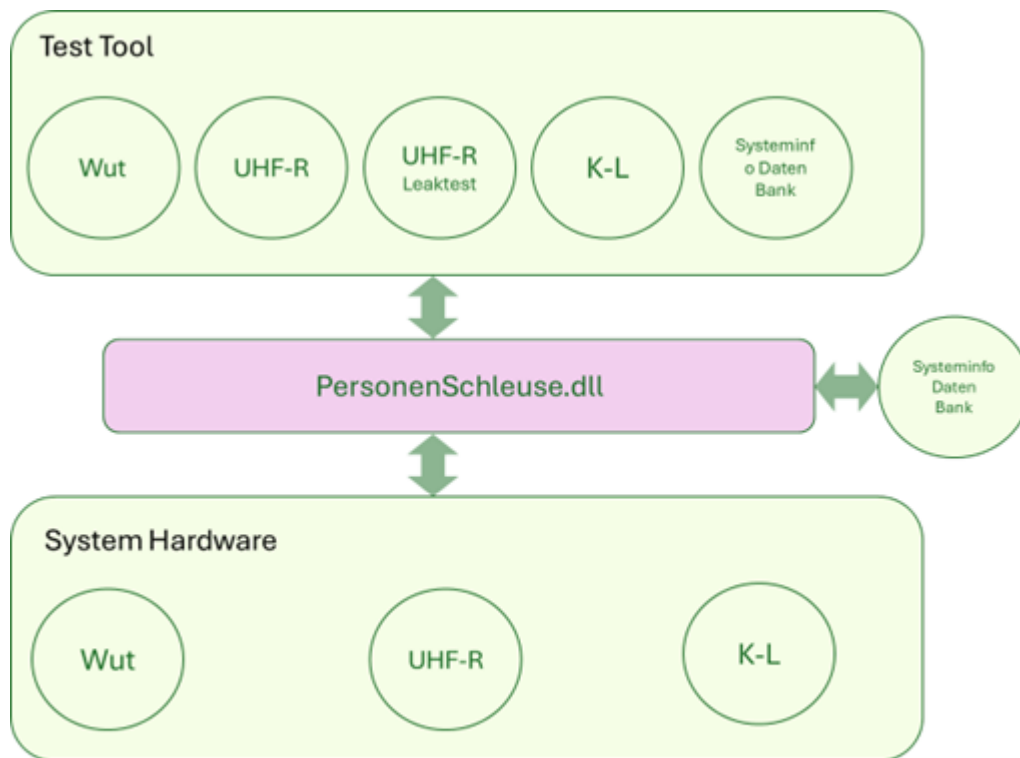
Bild5: Systemarchitektur-Diagramm
