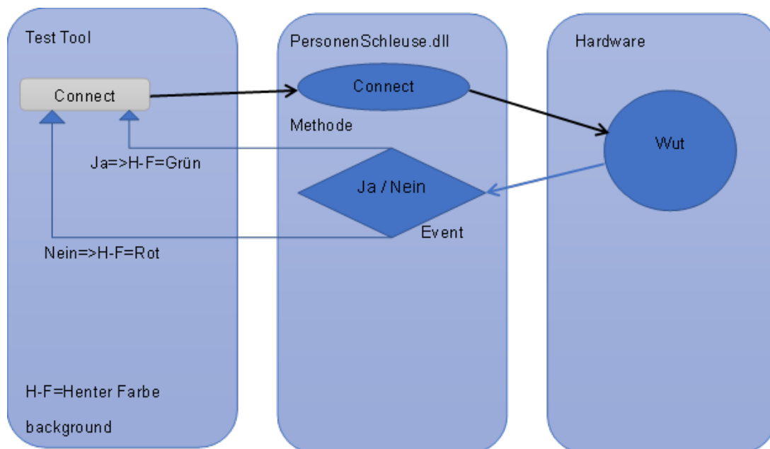
Bild 4: connect(uml)
