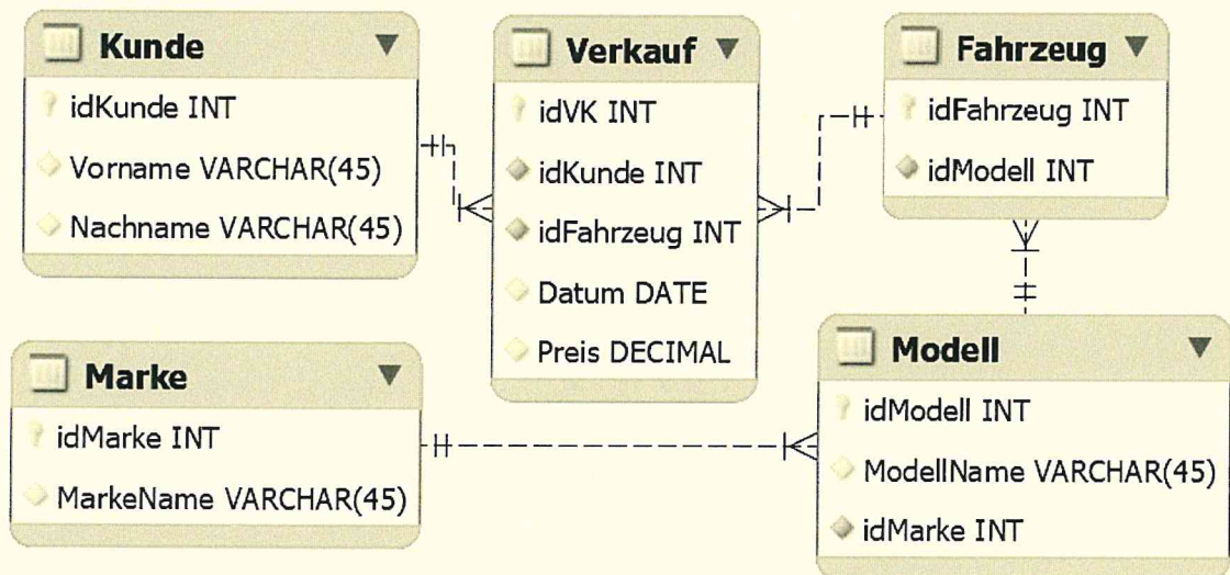
Abbildung 2: Datenmodell
